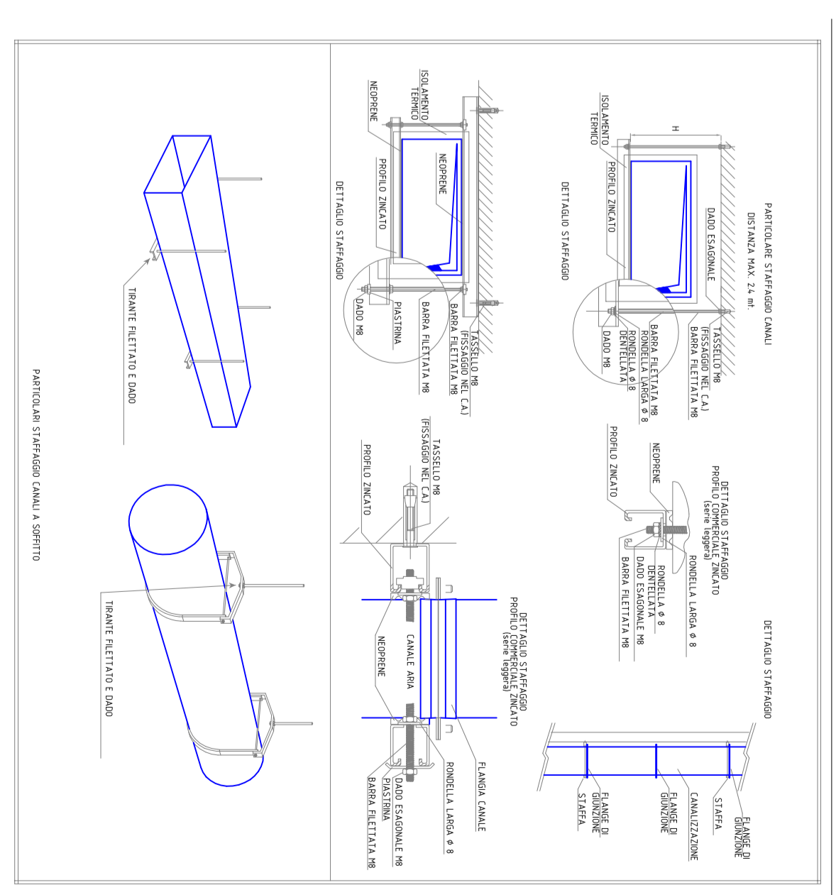
PARTICOLARE STAFFAGGIO CANALI RETTANGOLARI VERTICALI DISTANZA MASSIMA 2.400mm
